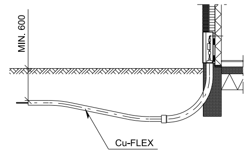
SNIT I HUSINDFØRING , 1:50 Cu-FLEX
