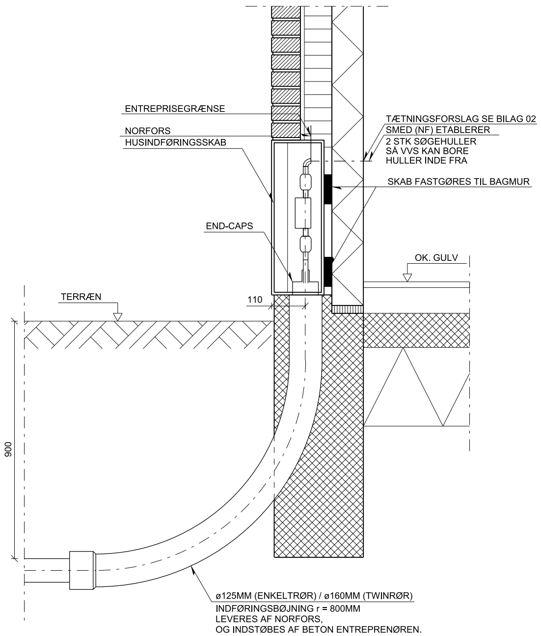
SNIT I HUSINDFØRING , 1:10 Cu-FLEX
