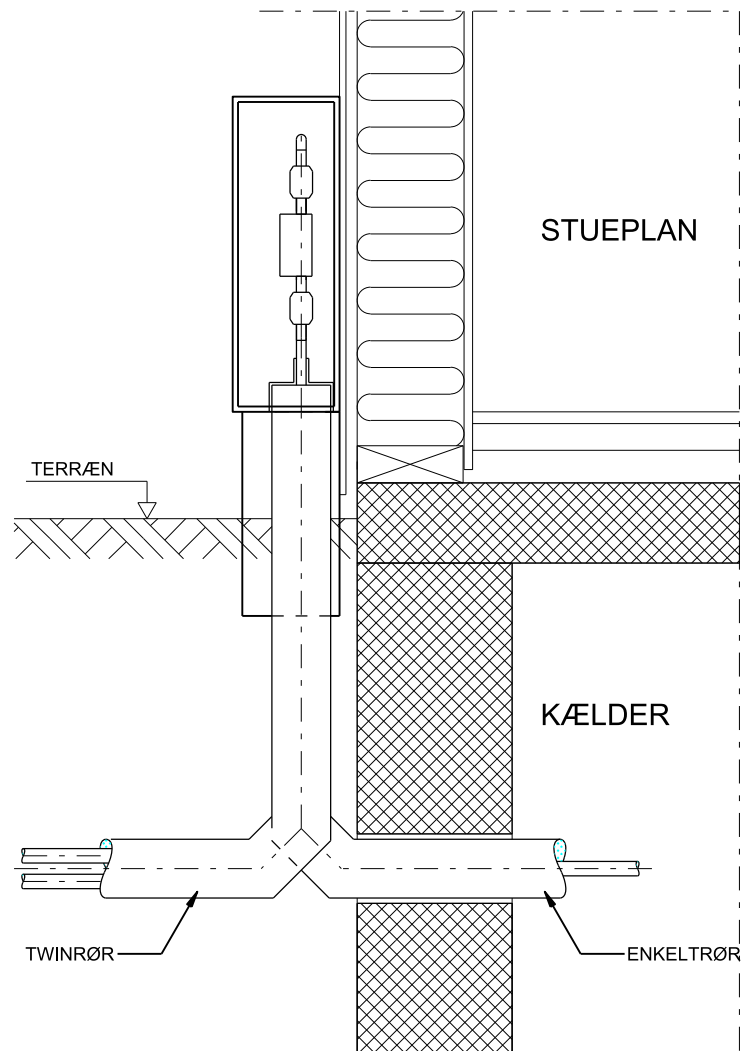
SNIT A-A , 1:10 Cu-FLEX TWIN OG ENKELTRØR
